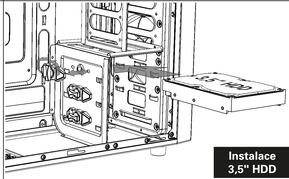
Instalace 3,5" jednotky
